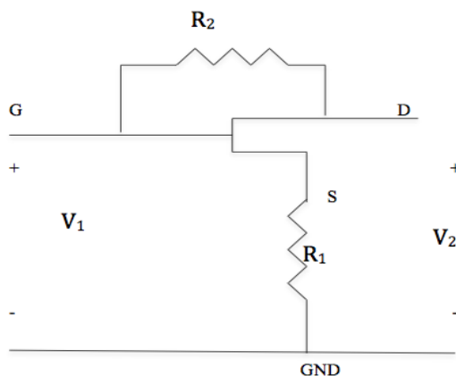
Fig. 8 BB Amplifier
