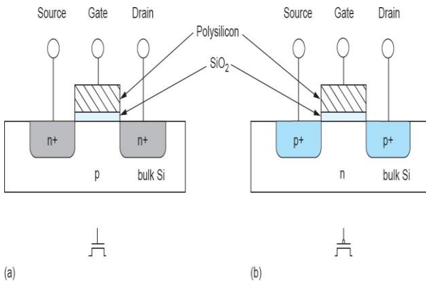
Fig. 3 a) n-MOS transistor b) p-MOS transistor
